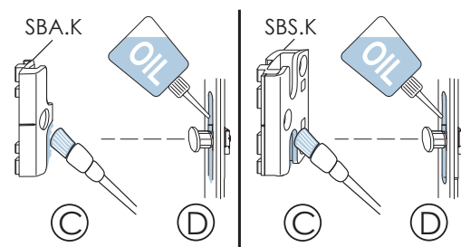
Dibujo 2: compás
