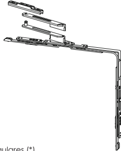
Conjunto de Angulares (*) Ref. 0301-EI (Izquierda) Ref. 0301-ED (Derecha)
